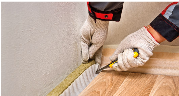
Рис. 14. Подрезка звукоизоляционных плит по периметру на уровне чистого пола
